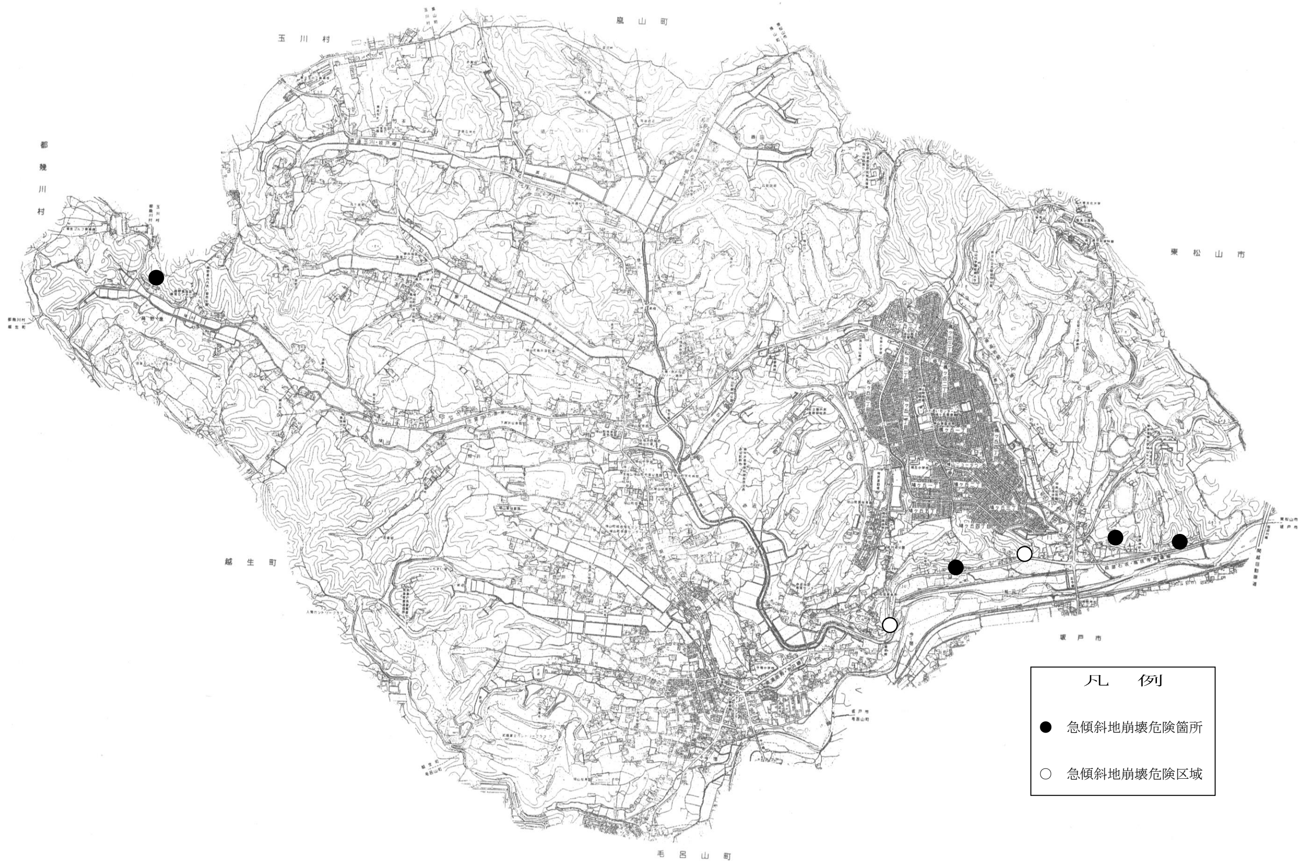
图 1-2-1 急傾斜地崩壊危険箇所・区域 (急傾斜地法)
