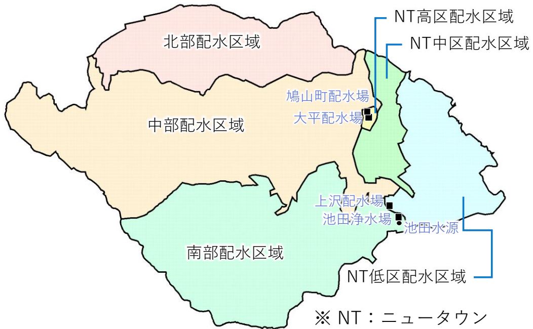
図 2-2 給水区域と施設配置
