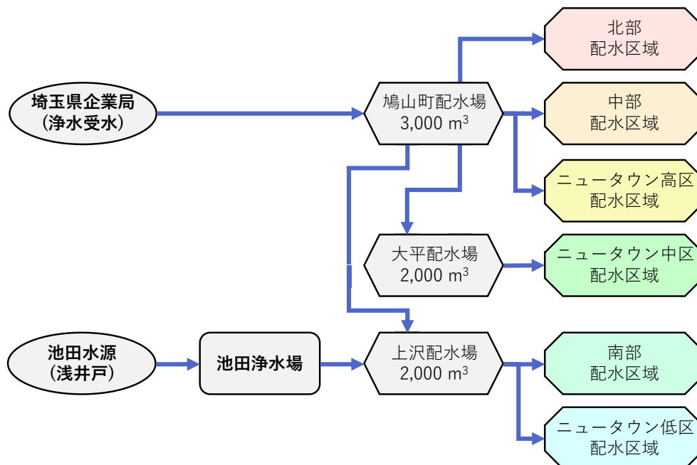
図 2-3 配水フロー
